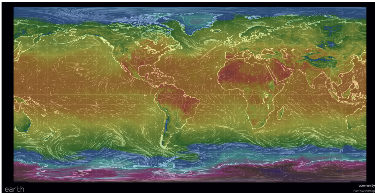
Figura 15: Direção do vento (traços) e Temperatura de Superfície (cor) em projeção equirretangular. Fonte: EarthWindMap
