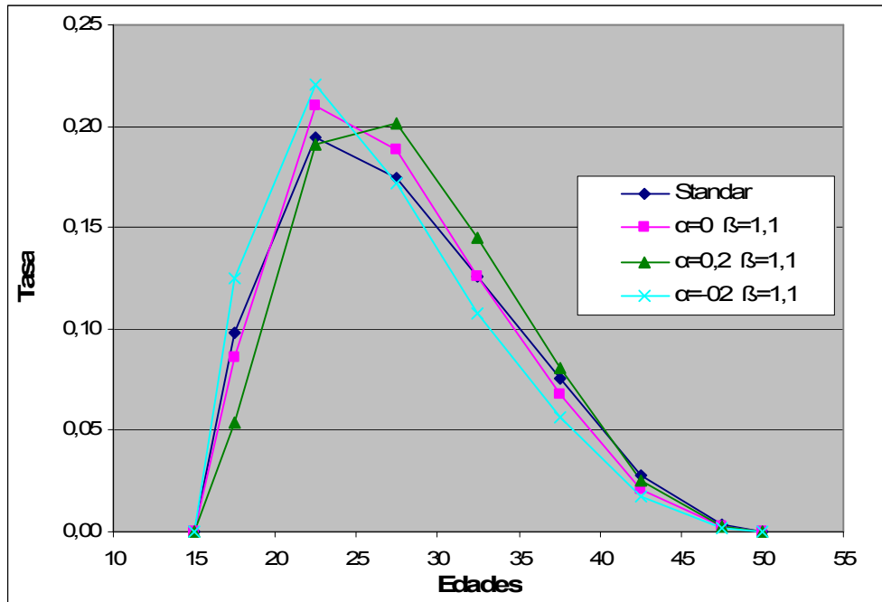
Gráfico 13. Estructuras teóricas de fecundidad derivadas con una estructura estándar y diversos valores de \alpha y \beta
