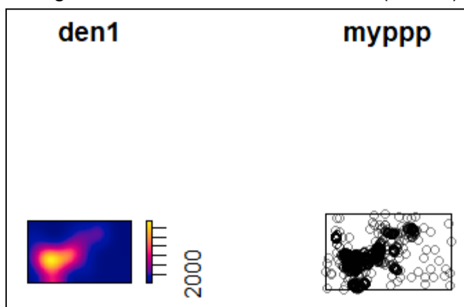
Imagem 2 - Estimativa de densidade (Kernel)
