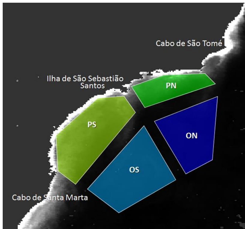
Figura 3: Divisão da área de estudo em quatro regiões, de acordo com os processos oceanográficos locais.
