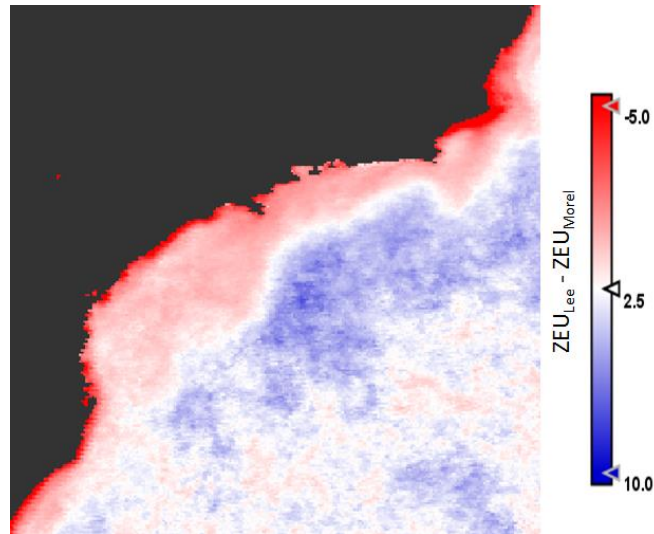
Figura 10: Diferença entre as profundidades da zona eufótica estimadas pelo modelo de Lee et al., (2007) e Morel et al., (2007). Regiões em azul a ZEU_{Lee} é maior que a ZEU_{Morel} . Regiões em vermelho a ZEU_{Lee} é menor que a ZEU_{Morel} .
