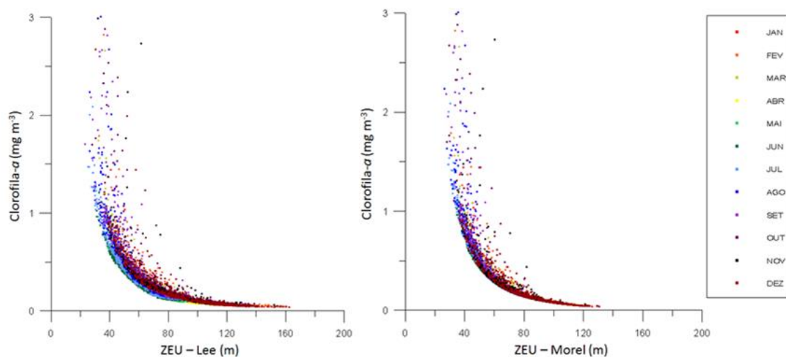
Figura 15: Correlação da CSM em função da ZEU. As cores estão associadas a diferentes meses do ano. Os valores plotados são as somas de todos os obtidos dos quatro polígonos definidos a priori.
