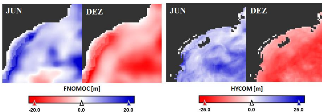
Figura 14: Anomalias da PCM para os modelos FNMOC (esquerda) e HYCOM (direita).
