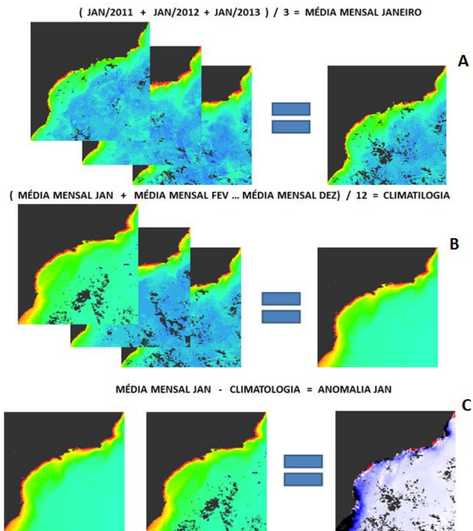
Figura 2: Pré-processamento dos produtos A) médias mensais, B) climatologia, C) anomalia, utilizados nas análises.
