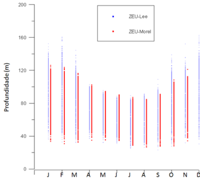
Figura 9: Distribuição temporal dos valores de ZEU_{Lee} e ZEU_{Morel} considerando os dados dentro dos 4 polígonos definidos a priori.
