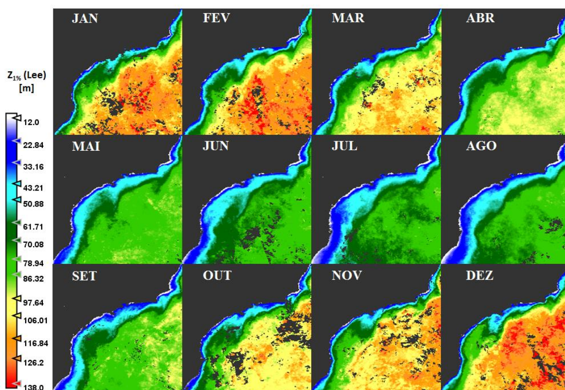
Figura 6: Zona eufótica estimada pelo modelo ZEU_{Lee} .
