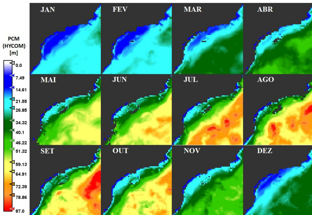
Figura 12: Profundidade da camada de mistura estimada pelo modelo HYCOM.
