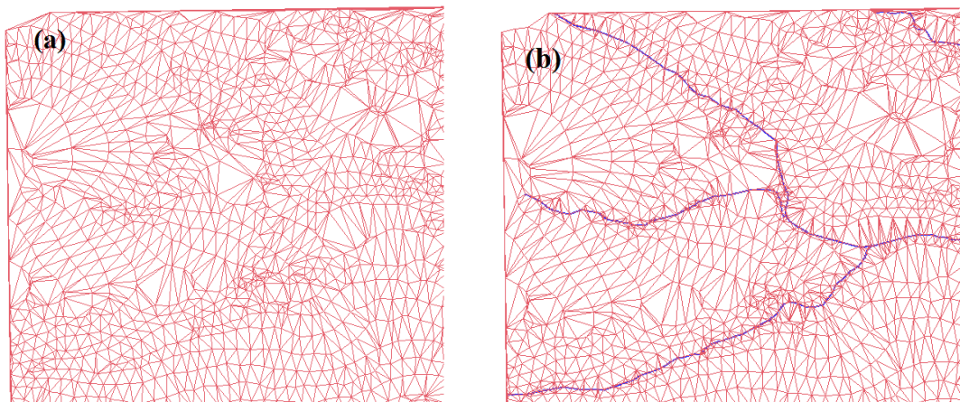
Figura 4: Grade triangular (TIN). Em (a) sem linha de quebra; (b) com linha de quebra.
