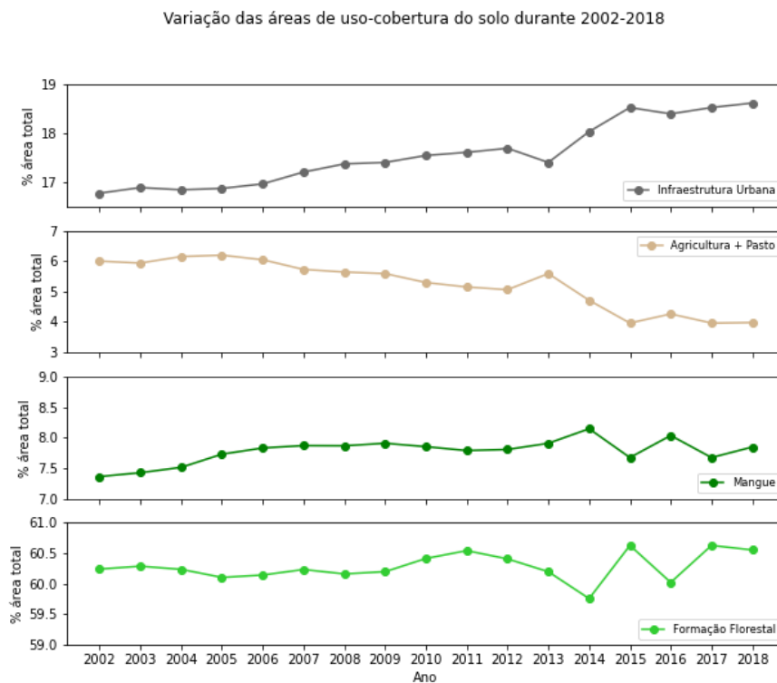
Figura 3.4 - Variação das áreas de uso-cobertura do solo sobre o Polo Central BHBS durante 2002-2018 considerando as classes de infraestrutura urbana (em cinza); agricultura e pasto (em bege); mangue (em verde escuro) e formação florestal (em verde claro).
