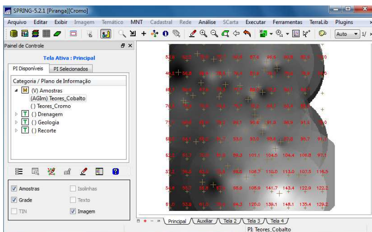
Figura 2: Grade Retangular a partir das amostras do PI “Teores_Cobalto”.
