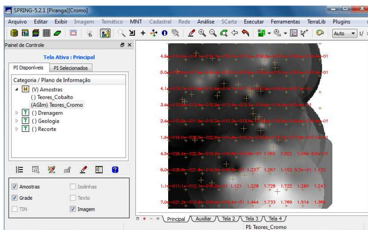
Figura 1: Grade Retangular a partir das amostras do PI “Teores_Cromo”.
