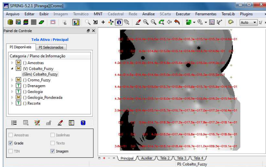
Figura 5: Teores de Cobalto classificado pelo método Fuzzy. Os valores variam de 0 (preto) até 1 (branco).
