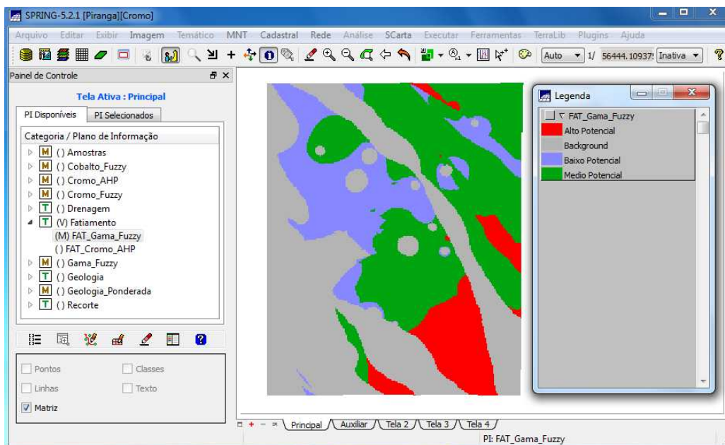
Figura 8: Mapas de Potencialidade de Cromo gerado pela Fuzzy Gama.
