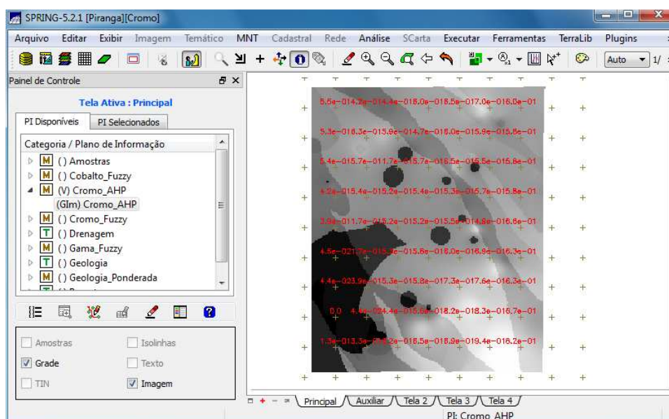
Figura 7: Cruzamento pela técnica AHP.
