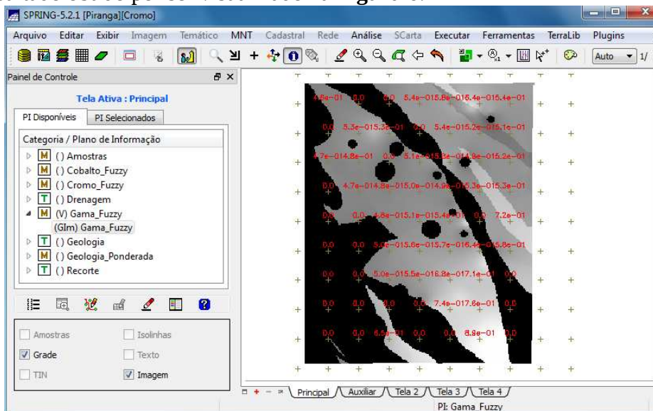
Figura 6: Cruzamento por Fuzzy Gama.
