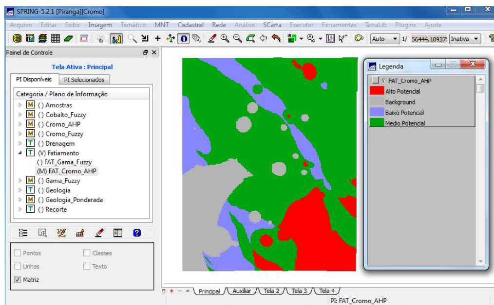
Figura 9: Mapas de Potencialidade de Cromo gerados pela técnica AHP.
