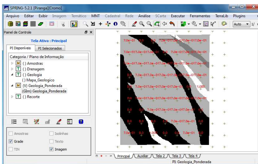
Figura 3: Mapa Ponderado da Geologia. As cores mais escuras representam o menor peso.
