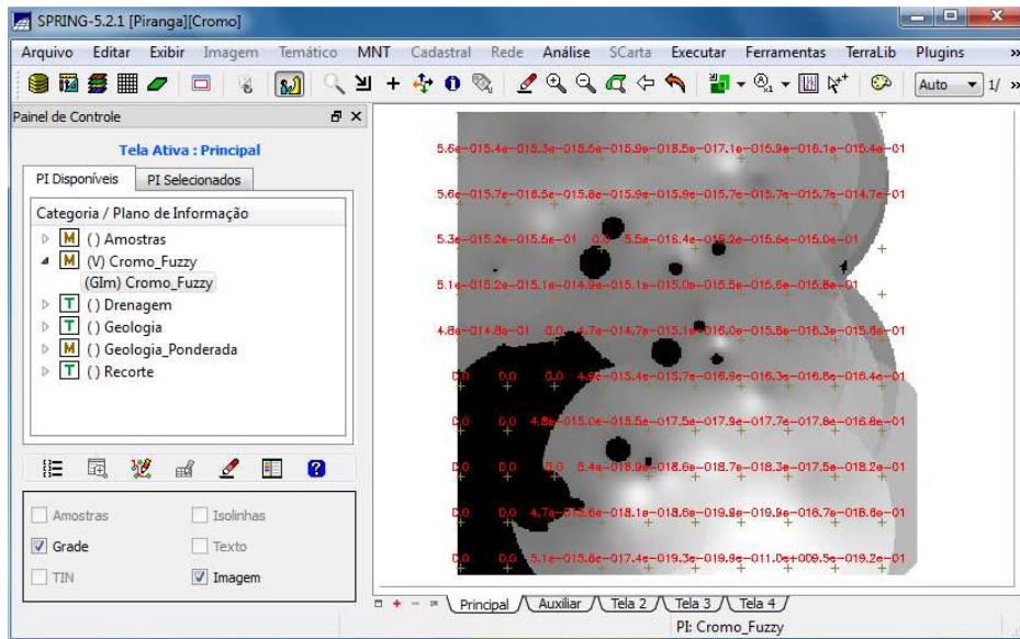
Figura 4: Teores de Cromo classificado pelo método Fuzzy. Os valores variam de 0 (preto) até 1(branco).
