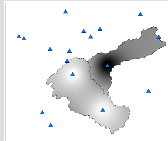
IDW
