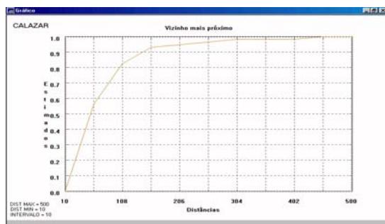
Figura 04. Análise univariada de pontos . Doença: CALAZAR, através do método do vizinho mais próximo, sendo Dmax= 500m; Dmin= 50m; t = 10m.
