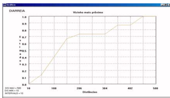
Figura 05. Análise univariada de pontos . Doença: DIARRÉIA, através do método do vizinho mais próximo, sendo Dmax= 500m; Dmin= 10m; t = 10m.
