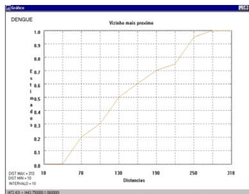
Figura 07. Análise univariada de pontos . Doença: DENGUE, através do método do vizinho mais próximo, sendo Dmax= 310; Dmin= 10; t = 10.
