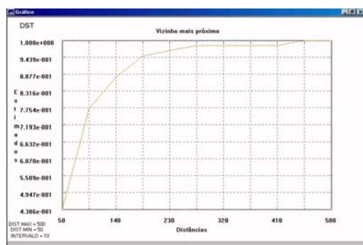
Figura 06. Análise univariada de pontos . Doença: DIARRÉIA, através do método do vizinho mais próximo, sendo Dmax= 500; Dmin= 50; t = 10.
