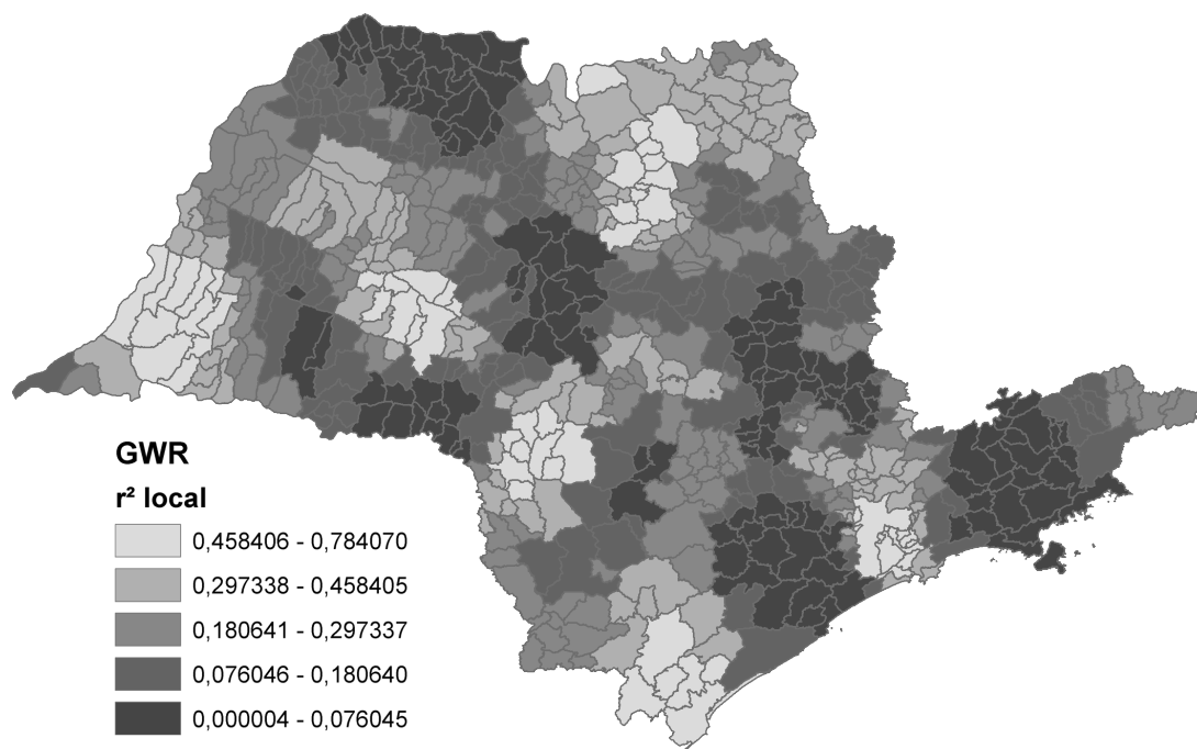
Figura 10: r^2 local ajustado para área de estudo
