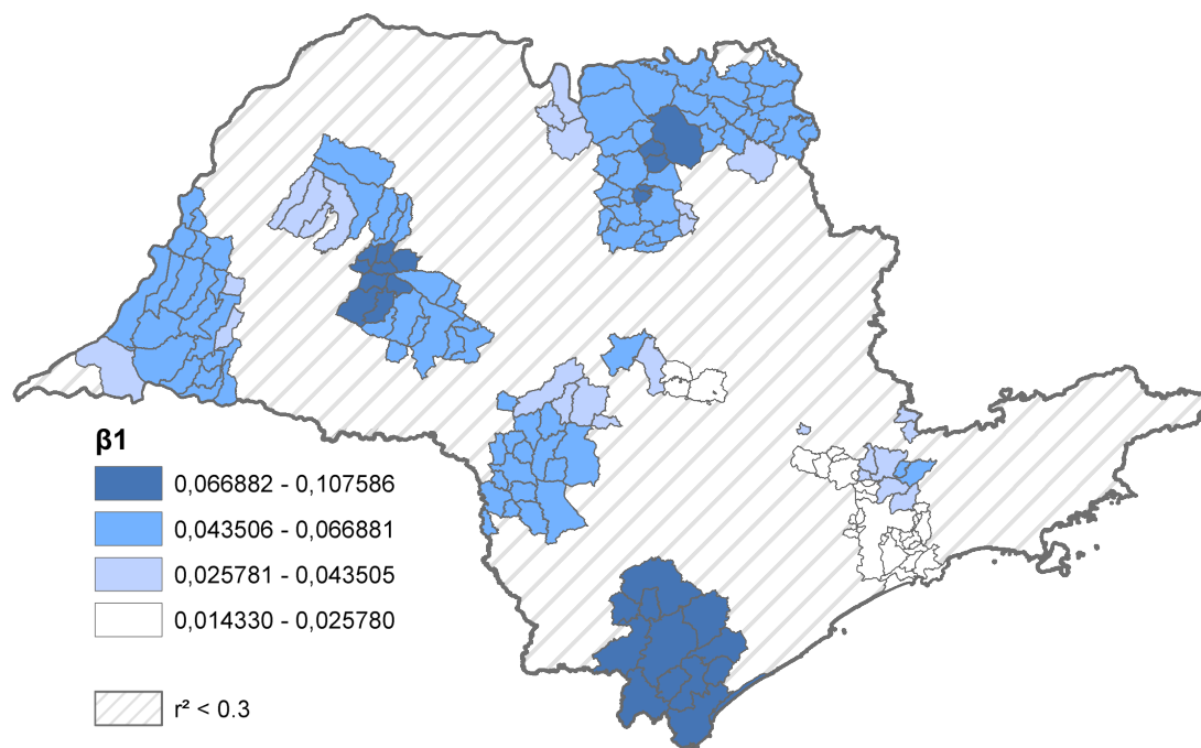
Figura 11: Áreas previstas onde o coeficiente angular é estimado sob r^2 superior a 0,3
