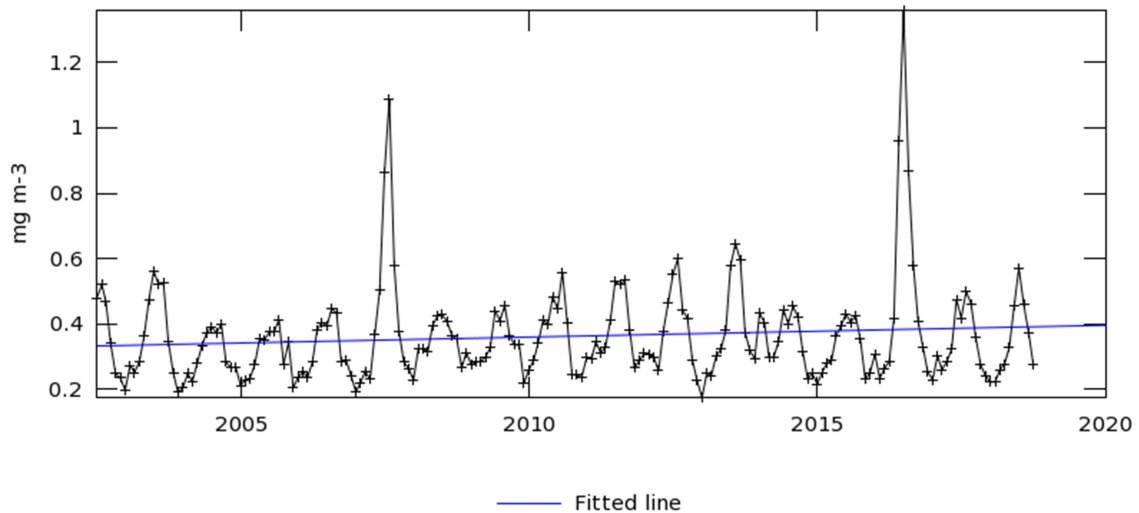
Figura 6 – Média dos valores mensais da concentração de clorofila-a ( \text{mg}/\text{m}^3 ) na região da Bacia de Santos com linha ajustada para o período de janeiro de 2002 a novembro de 2018.
