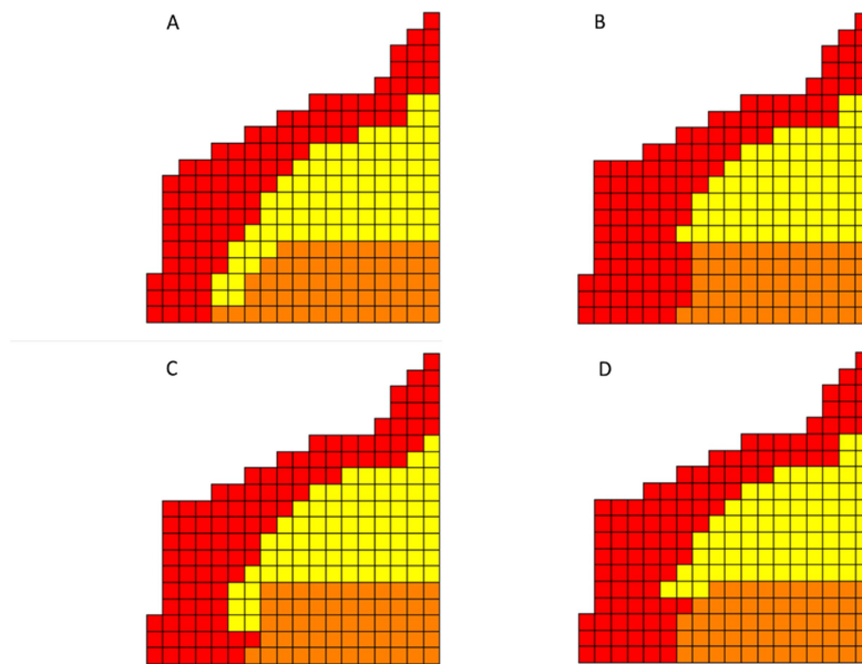
Figura 7 – Regionalização da região da Bacia de Santos utilizando o algoritmo SKATER por média sazonal. A - Verão, B - Outono, C - Inverno, D - Primavera. Para o período de janeiro de 2002 a novembro de 2018.
