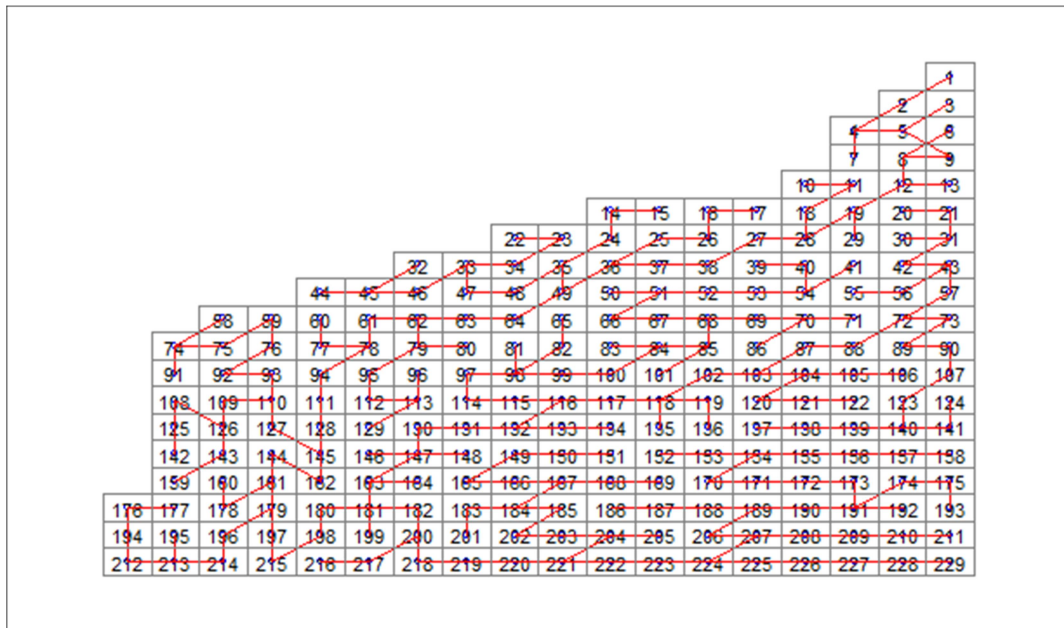
Figura 2 – Exemplo de árvore geradora mínima (média do verão).
