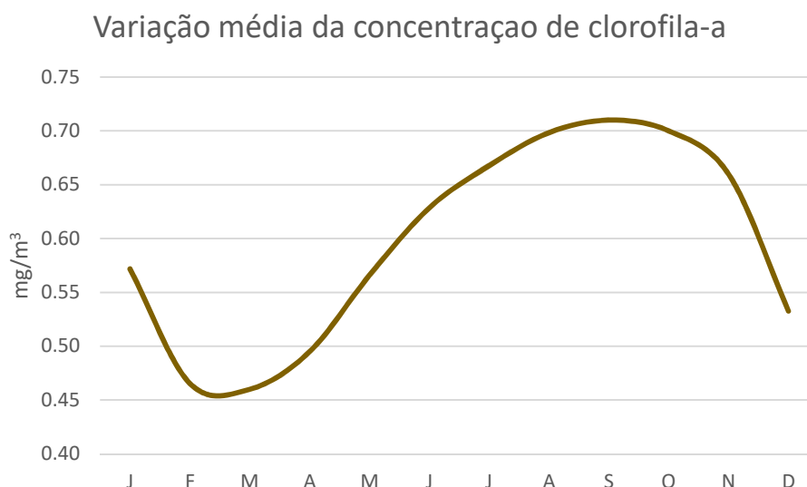
Figura 4 – Valores médios agrupados por mês de concentração de clorofila-a ( \text{mg}/\text{m}^3 ) para o período de setembro de 1997 a novembro de 2018.
