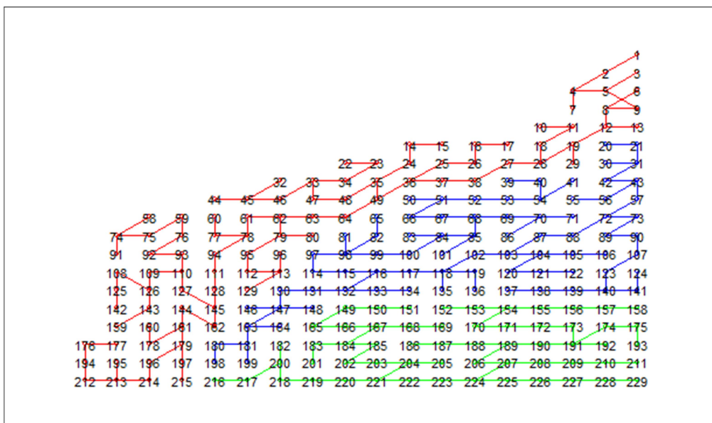
Figura 3. Exemplo de agrupamento de geo-objetos com características semelhantes (média do verão).
