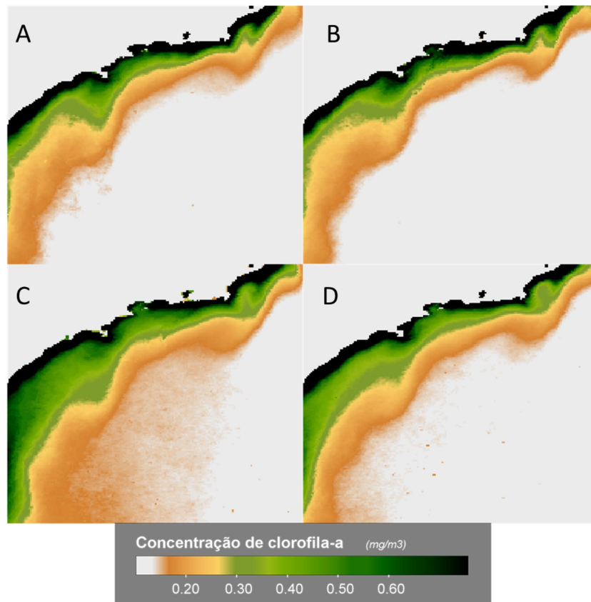
Figura 5 - Concentração de clorofila-a ( \text{mg/m}^3 ) na região da Bacia de Santos por média sazonal. A - Verão, B - Outono, C - Inverno, D – Primavera costeira para o período de setembro de 1997 a novembro de 2018.
