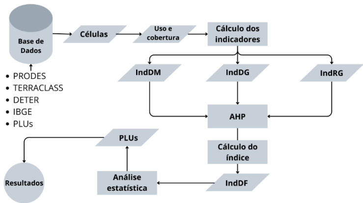
Figura 3. Fluxograma Metodológico
